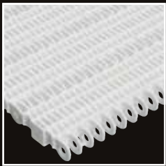
50-401 Superficie muy abierta. Máximo caudal de aire en enfriado y congelado
