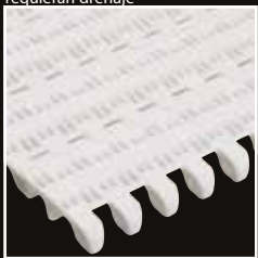
50-806 Superficie plana perforada fácil de limpiar en aplicaciones que requieren un simple drenaje.
