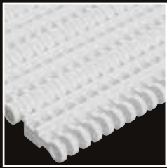
50-300 Superficie de pailla abierta para drenaje. Bajo contacto del producto con mayor agarre para producto congelado o ligeramente inclinado
