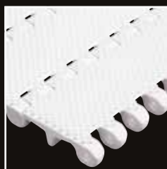
50-838 Superficie cerrada plana con múltiples puntos para disminuir el contacto con productos pegajosos. Fácil limpieza.
