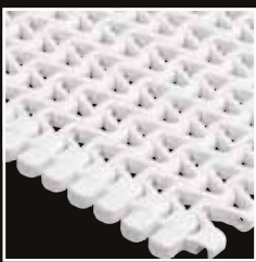
12-401 Módulo redondeado y muy abierto. Máximo caudal de aire para aplicaciones de secado. Limpieza muy fácil
